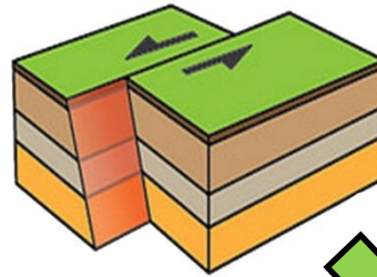
รอยเลื่อนตามแนวระดับแบบเหลื่อมซ้าย (left lateral strike slip fault)
