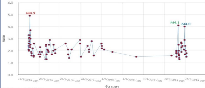
แผ่นดินไหววังเหนือ จ.ลำปาง ระหว่างวันที่ 20 กุมภาพันธ์ - 15 มีนาคม 2562
