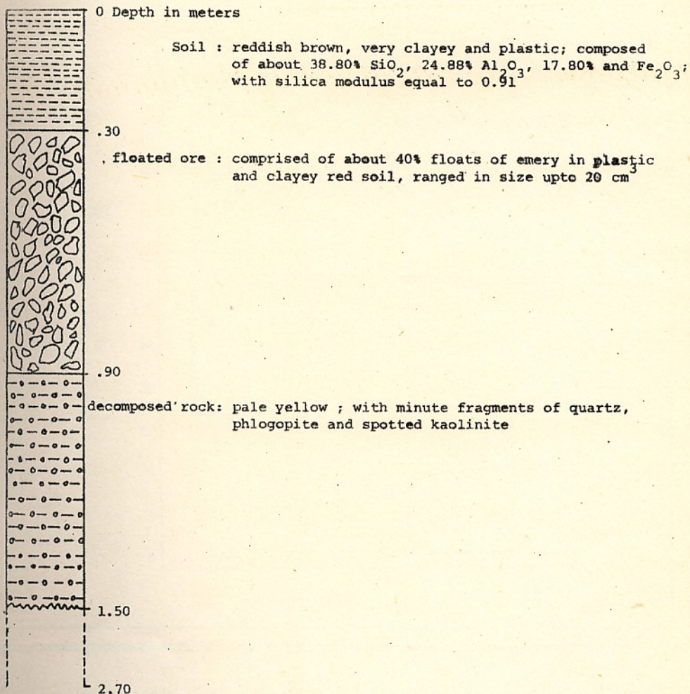
รูปที่ ๖. แสดงลักษณะของชั้นดินและชั้นแร่ก่อนชนิด float ore ในหลุมขุด P 2 ของแหล่งแร่ A บริเวณเนินผู้ใหญ่ - พรหมา บ้านยุบธิปูน ต.ตะขบ อ.ปรางค์ไทย จ.นครราชสีมา
