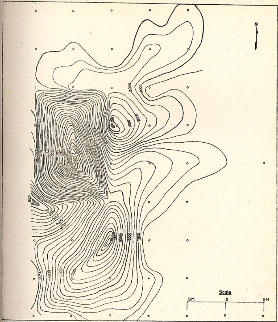
แผนที่ ๔. แผนที่แสดงค่าความเข้มสนามแม่เหล็กโลกในแนวตั้ง บริเวณแหล่งแร่ C ทางตอนเหนือ (CN) ของเส้นทางที่ผ่านที่ตั้งบริษัทรับซื้อข้าวโพด บ้านยุบฮินัน ด.ตะขบ อ.ปรางค์ไทย จ.นครราชสีมา contour interval 1000 gamma
