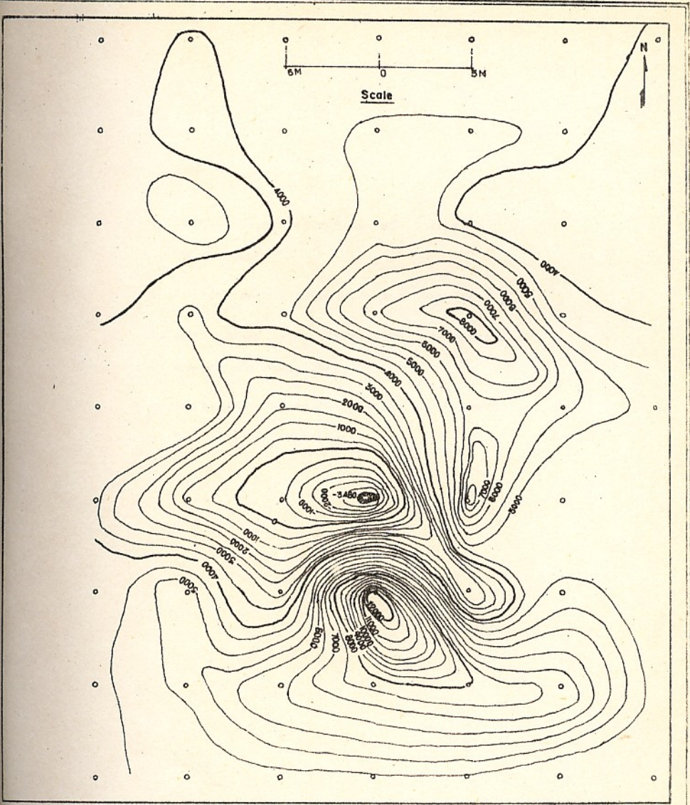
๑๐. แผนที่แสดงค่าความเข้มของสนามแม่เหล็กโลกในแนวตั้ง บริเวณแหล่งแร่ C ทางตอนใต้ (CS) ของเส้นทางที่ผ่านที่ตั้งบริษัทรับซื้อข้าวโพด บ้านยุบยี่ปุ่น ต.ตะขบ อ.ปรางค์กู่ จ.นครราชสีมา contour interval 1000 gamma
