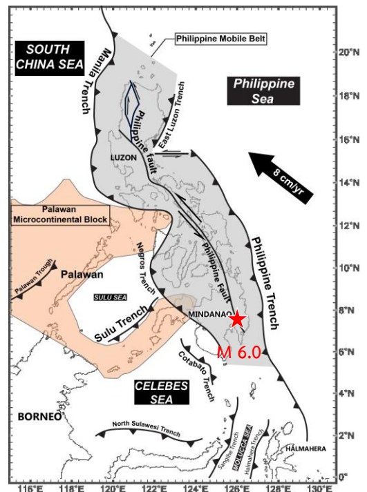
แผนที่แสดงรอยเลื่อน Philippine fault zone
