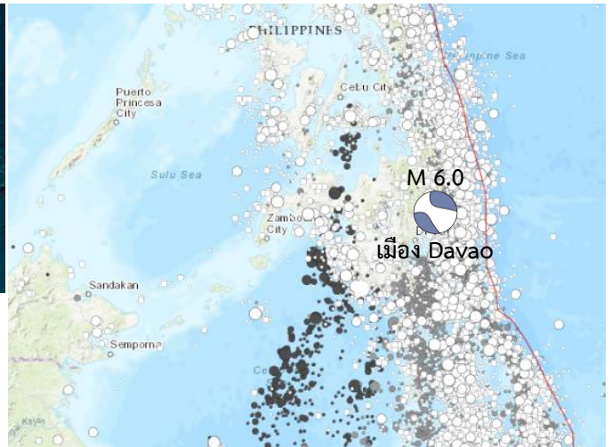
แผนที่แสดงจุดเหนือศูนย์เกิดแผ่นดินไหวบนบก ขนาด 6.0 ประเทศฟิลิปปินส์ (ที่มา : USGS)
