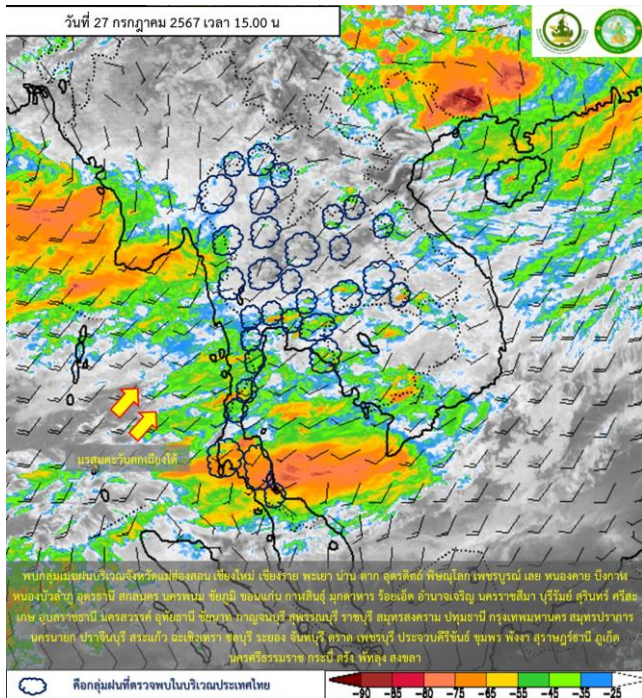
ภาพถ่ายดาวเทียม วันที่ 27 ก.ค. 67 เวลา 15.00 น. (ที่มา : กรมอุตุนิยมวิทยา)
